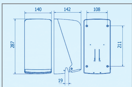
AF50000
