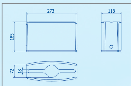
AH52000
