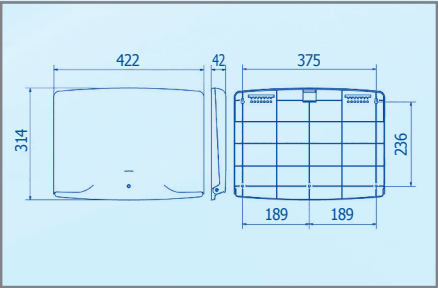
Dimensiones embalaje: (mm) 338 Packaging dimensions: 430 52
