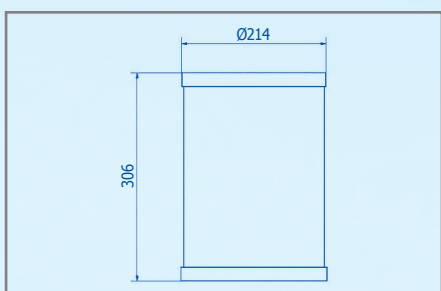
AL60000
