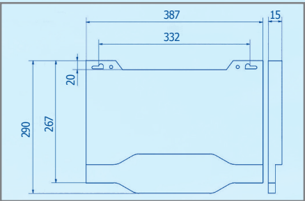
Dimensiones embalaje: (mm) 320 Packaging dimensions: 410 135
